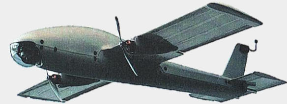
Комплекс с БпЛА ближнего действия «Молния-2Р»
